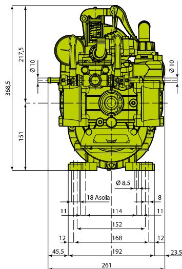
AR 30 GI 40 ET con CR 1:2,85 cod. 1624
